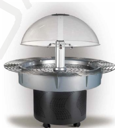
Okrogla hlajena vitrina Isola Dim. 1450x1310xh1560mm Za raznovrstna živila Temp. območje +3°C do +10°C Napetost 230V
