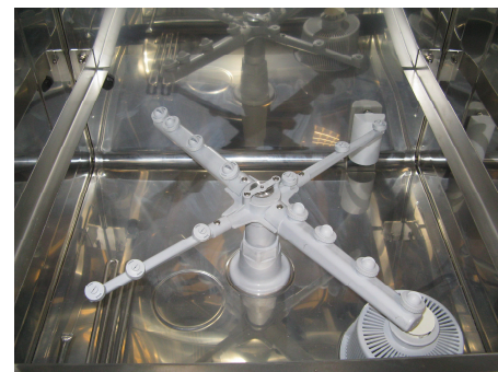
PVC pomivalne in izpiralne roke s prelivnim filtrom
